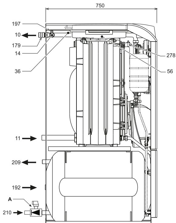
Vista lateral ATLAS D ECO 30 K
