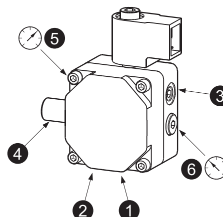
fig. 26- Bomba DANFOSS
