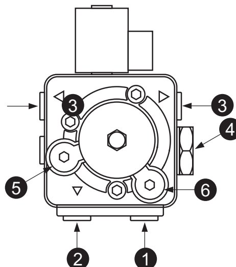
fig. 25- Bomba ITALPUMP
