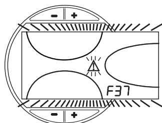
fig. 16 - Anomalia por baja presión en la instalación - Llave de llenado
